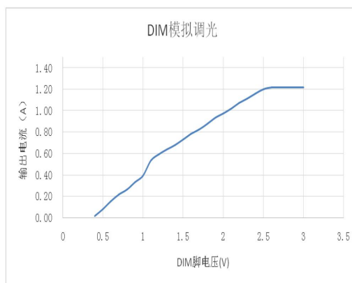
DIM 线性调光特性曲线
