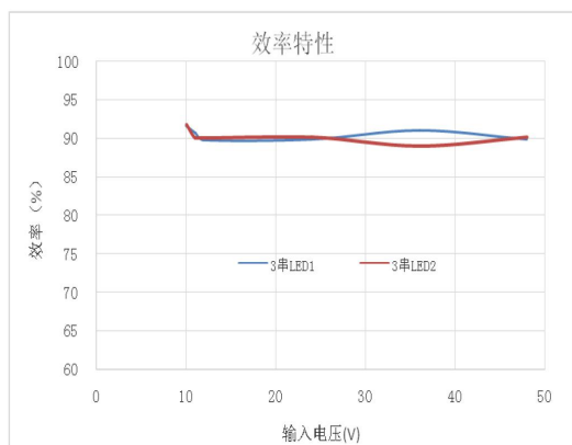
效率特性曲线
