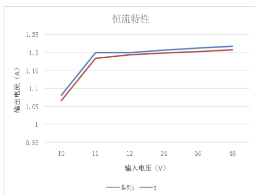
恒流特性曲线 (3 串 LED)
