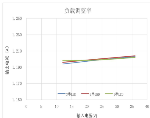
负载和母线调整率
