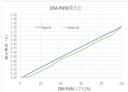
DIM 脚 PWM 调光特性曲线
